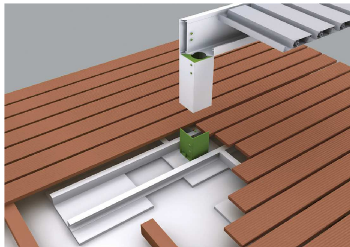
mocowanie na tarasie bez kotwienia
