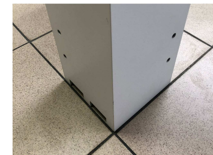
solidny stęp 15x15cm z odpływem wody w wybranym kierunku
