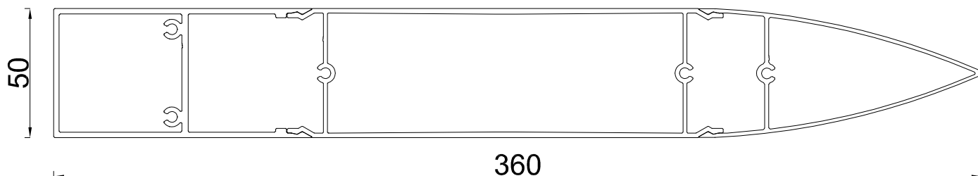
Zaślepka prosta
