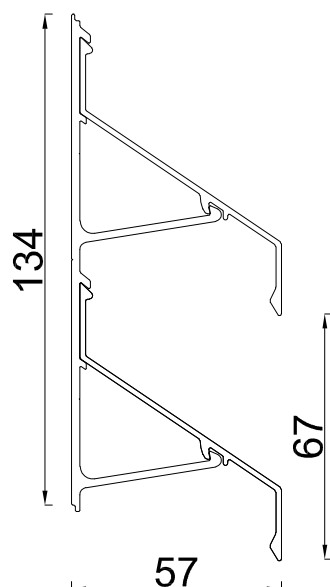
PROFIL ST 85C
