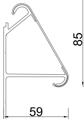
PROFIL ST 85C
