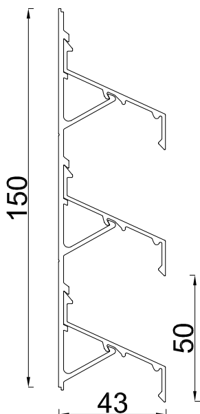
PROFIL ST 67Z
