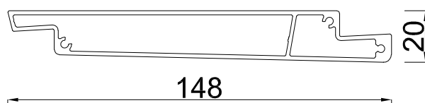
TYP145 BRISOLLEIL
