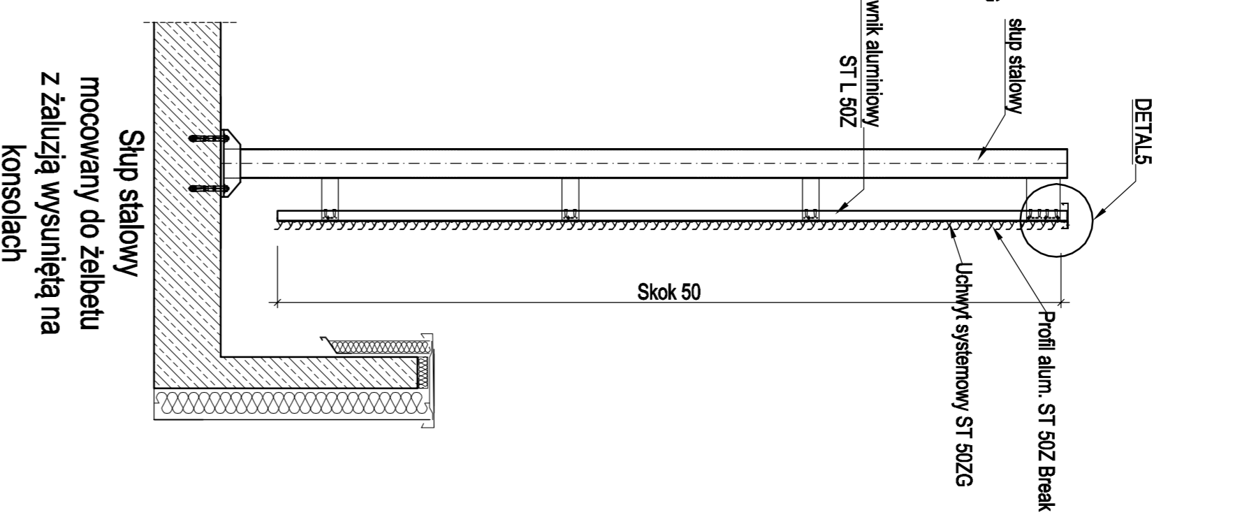
Przekrój pionowy wariant 1 skala 1:25
