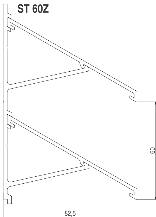
PROFIL ST 60Z GRZEBIEŃ ST 60ZG
