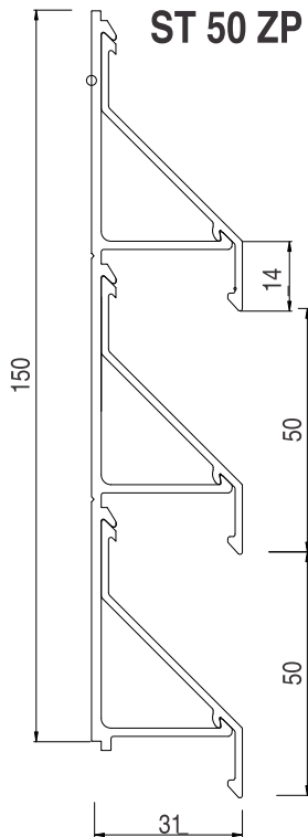
PROFIL ST 50ZP GRZEBIEŃ ST 50ZPG
