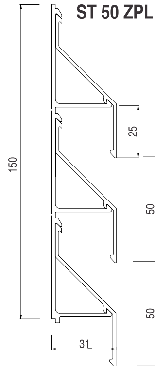
PROFIL ST 50ZPL GRZEBIEŃ ST 50ZPG
